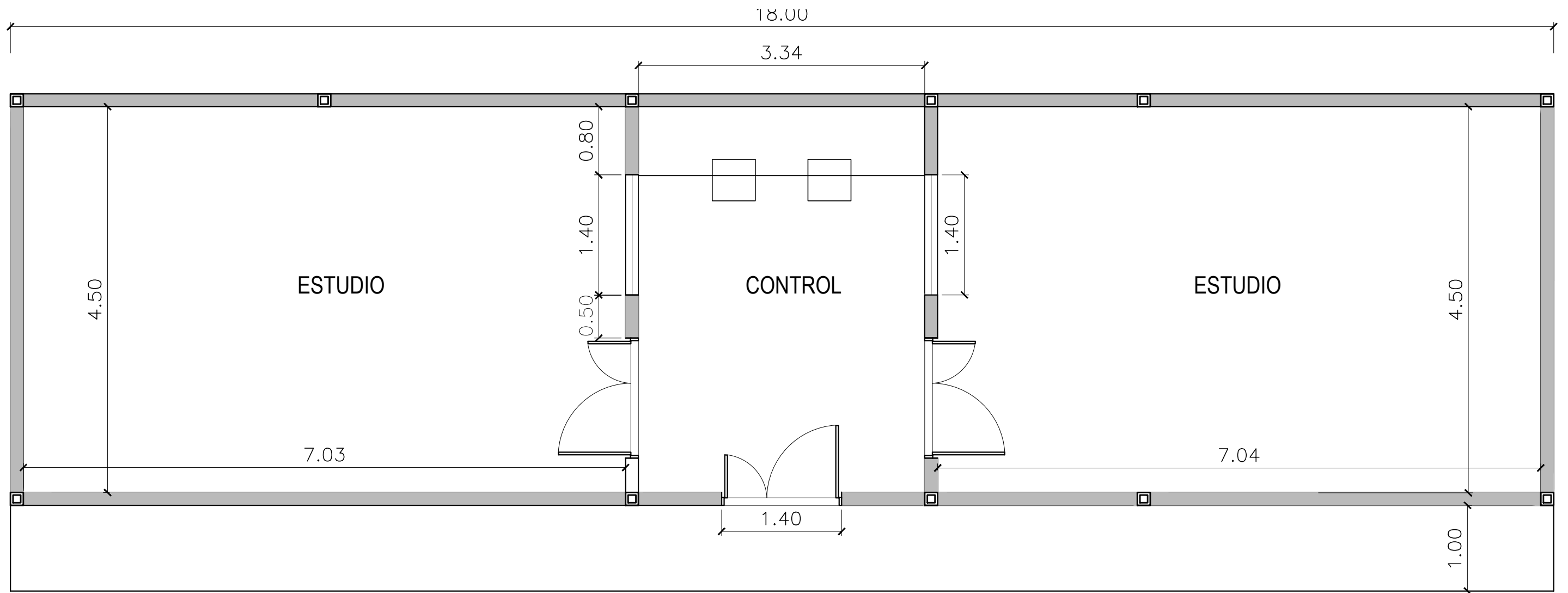
PLANTA ALTA
